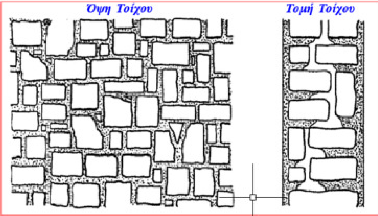
Βαθύ Αρμολόγημα
